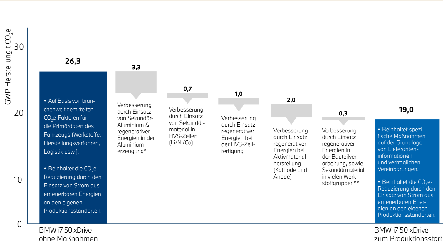
Abb. 5: Einfluss von Entwicklungszielen auf den Carbon Footprint der Herstellungsphase des BMW i7 50 xDrive.
